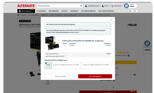
Nachher: Z-Index 1000
