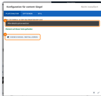
Content-Siegel: CSS-Selektor
